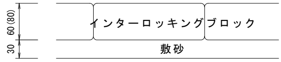
インターロッキングブロック
