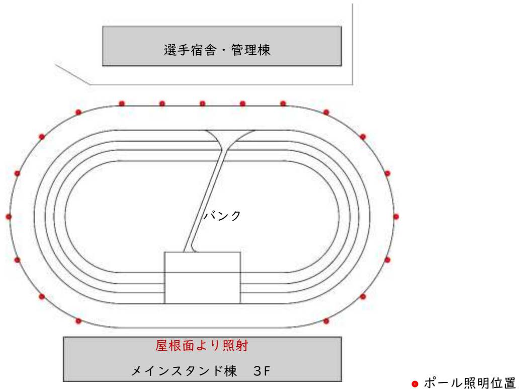
【図 5.14 バンク照明計画図】
