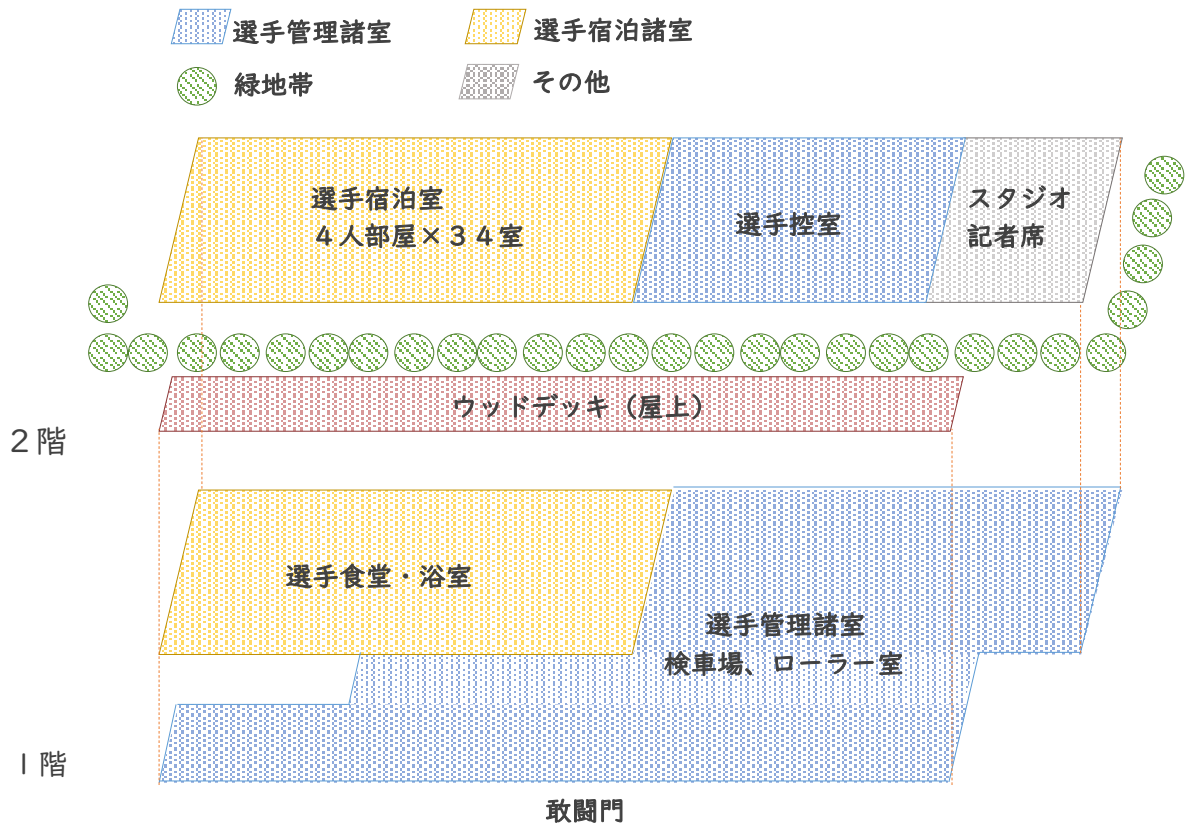
【図 5.9 選手宿舎・管理棟 平面図（図の下がバンク側）】
