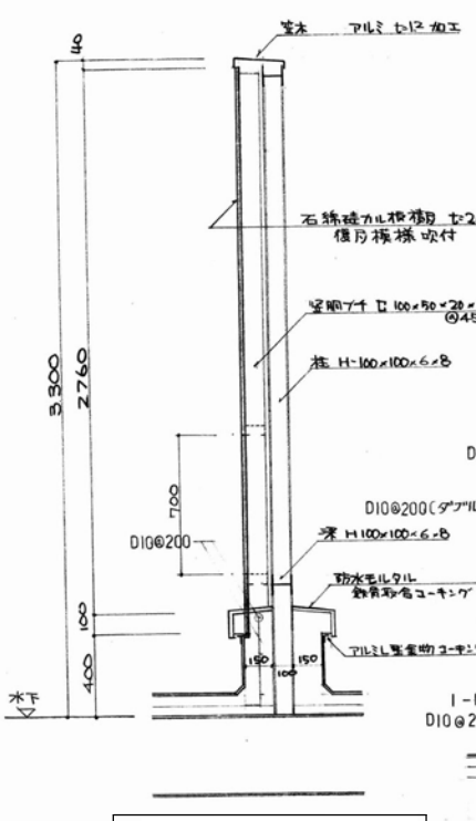
防音壁詳細図 S=1/30
