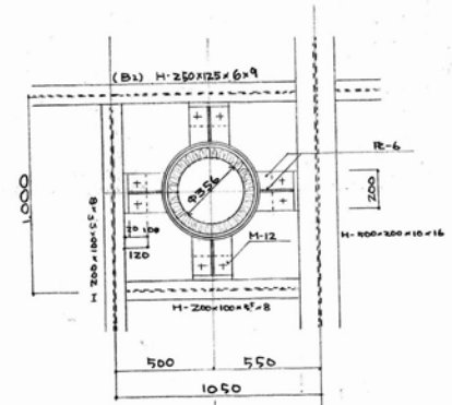
研修棟屋根鉄骨架台
