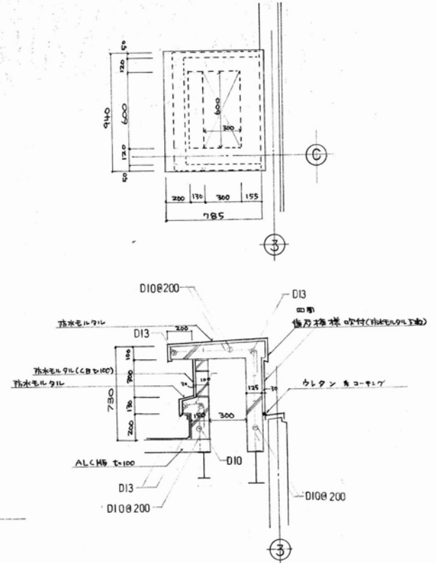
研修棟 P S立上り詳細図 S=1/30
