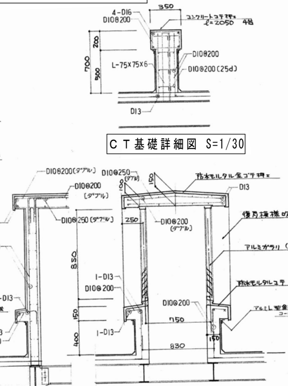
排気塔詳細図 S=1/30
