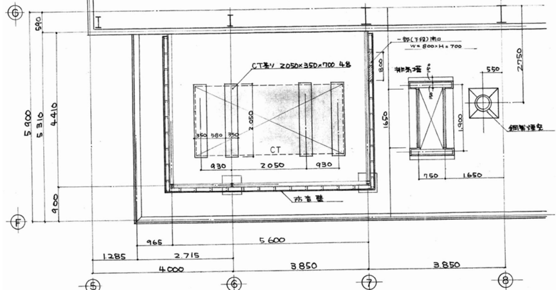
CT廻り平面詳細図 S=1/75
