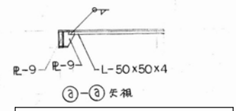
設備基礎詳細図 S=1/45
