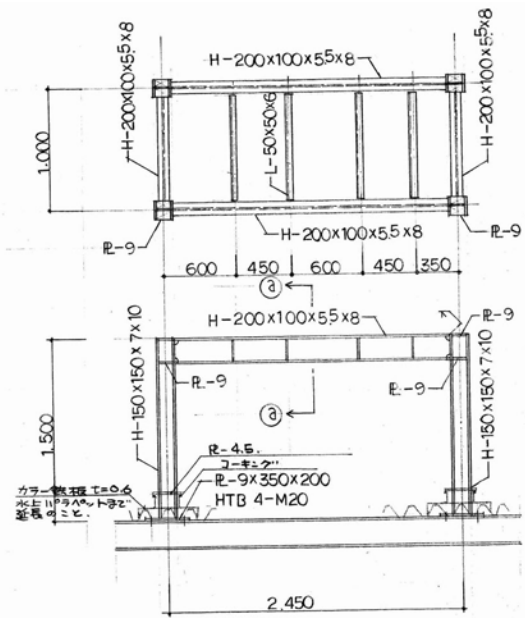
研修棟屋根鉄骨架台
