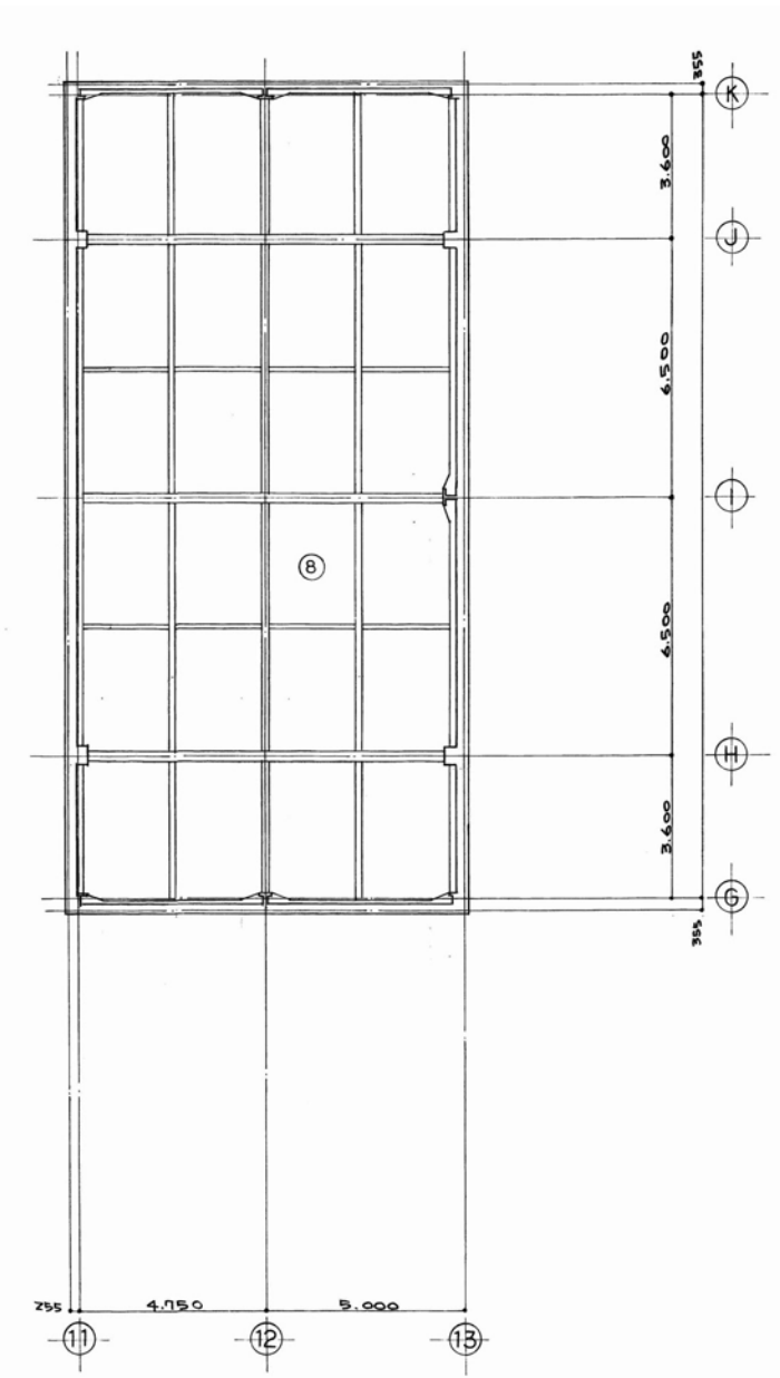
ステージ最上部 天井伏図 S=1/150
