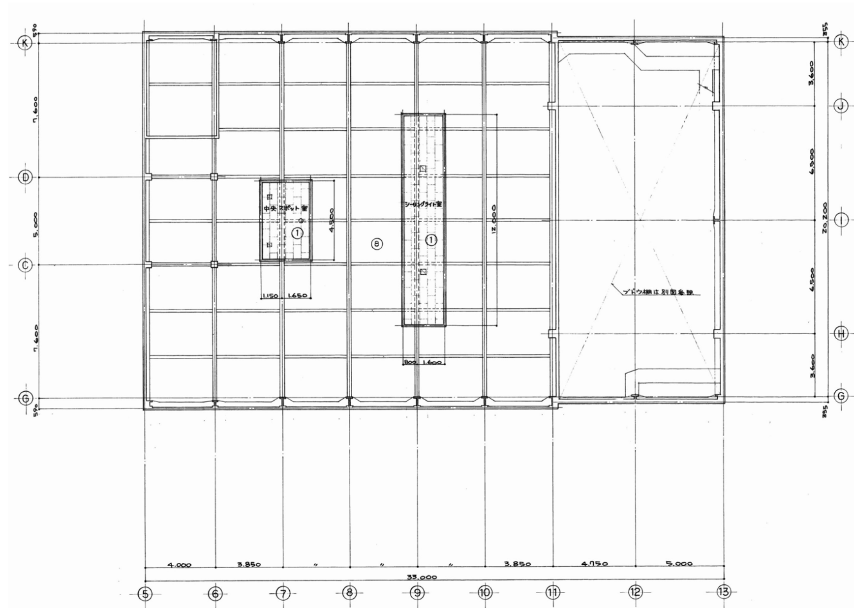
3階天井伏図 S=1/150
