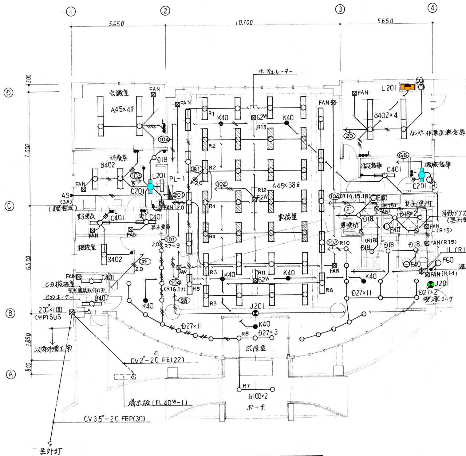
1階平面図 1/100
