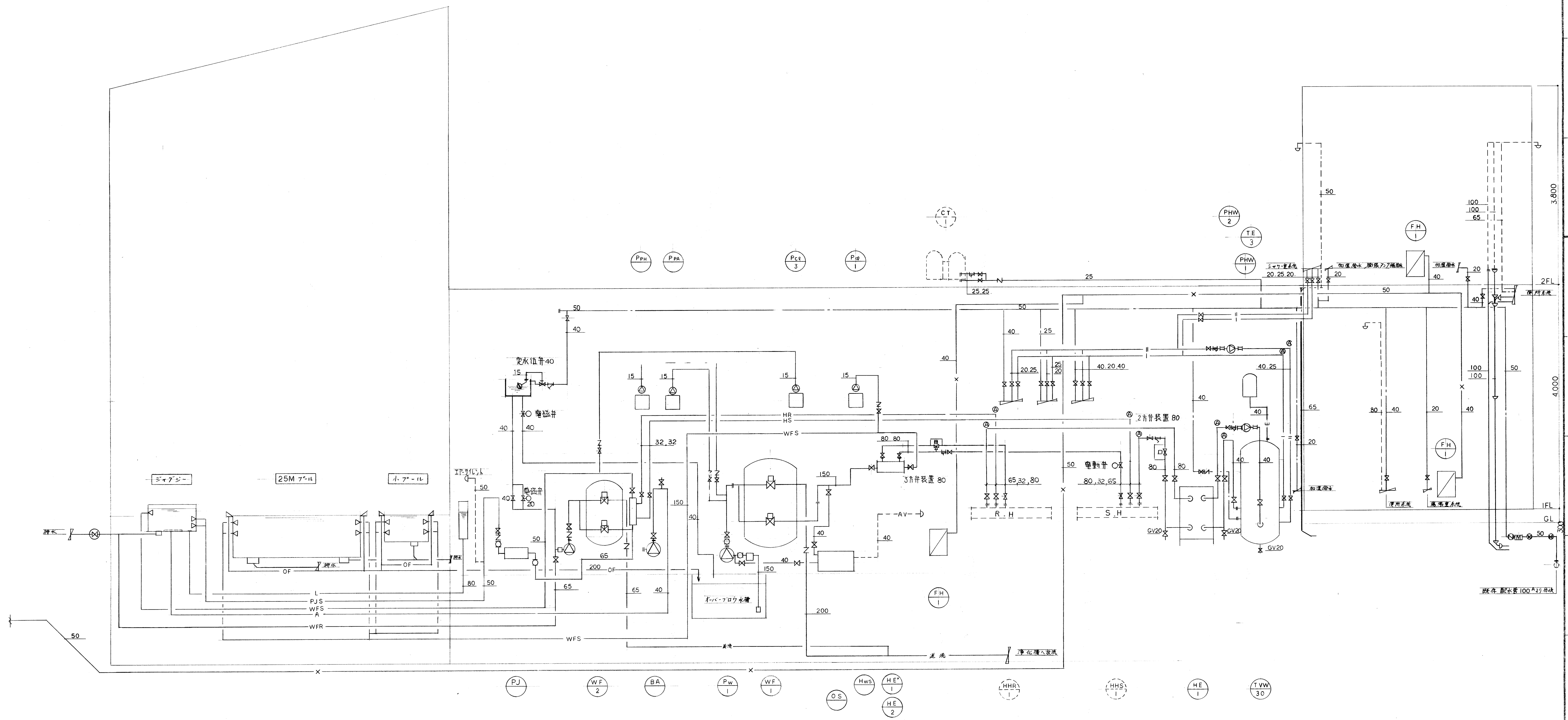
系統図(衛生)
