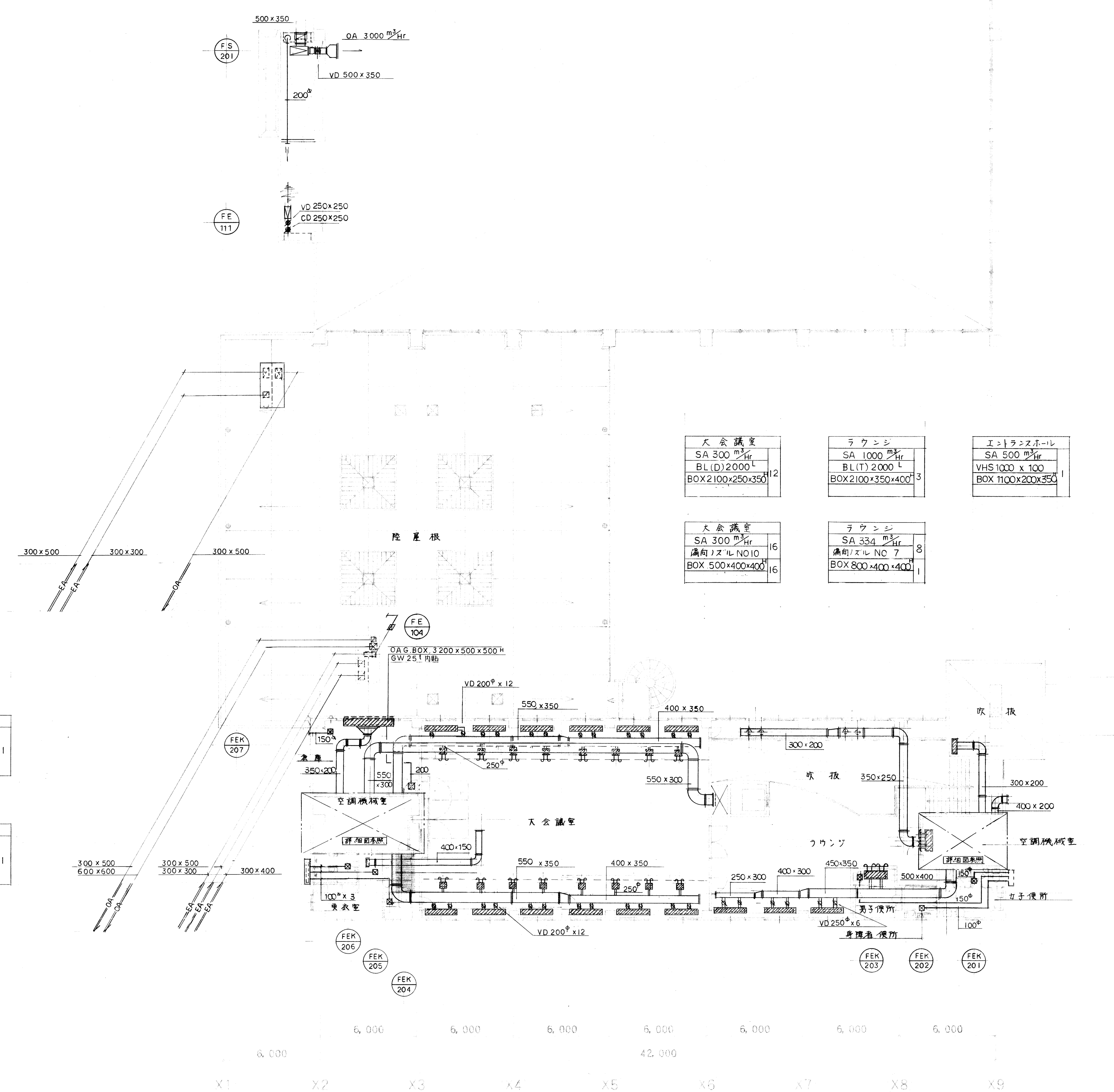
2階平面図 0=1/150
