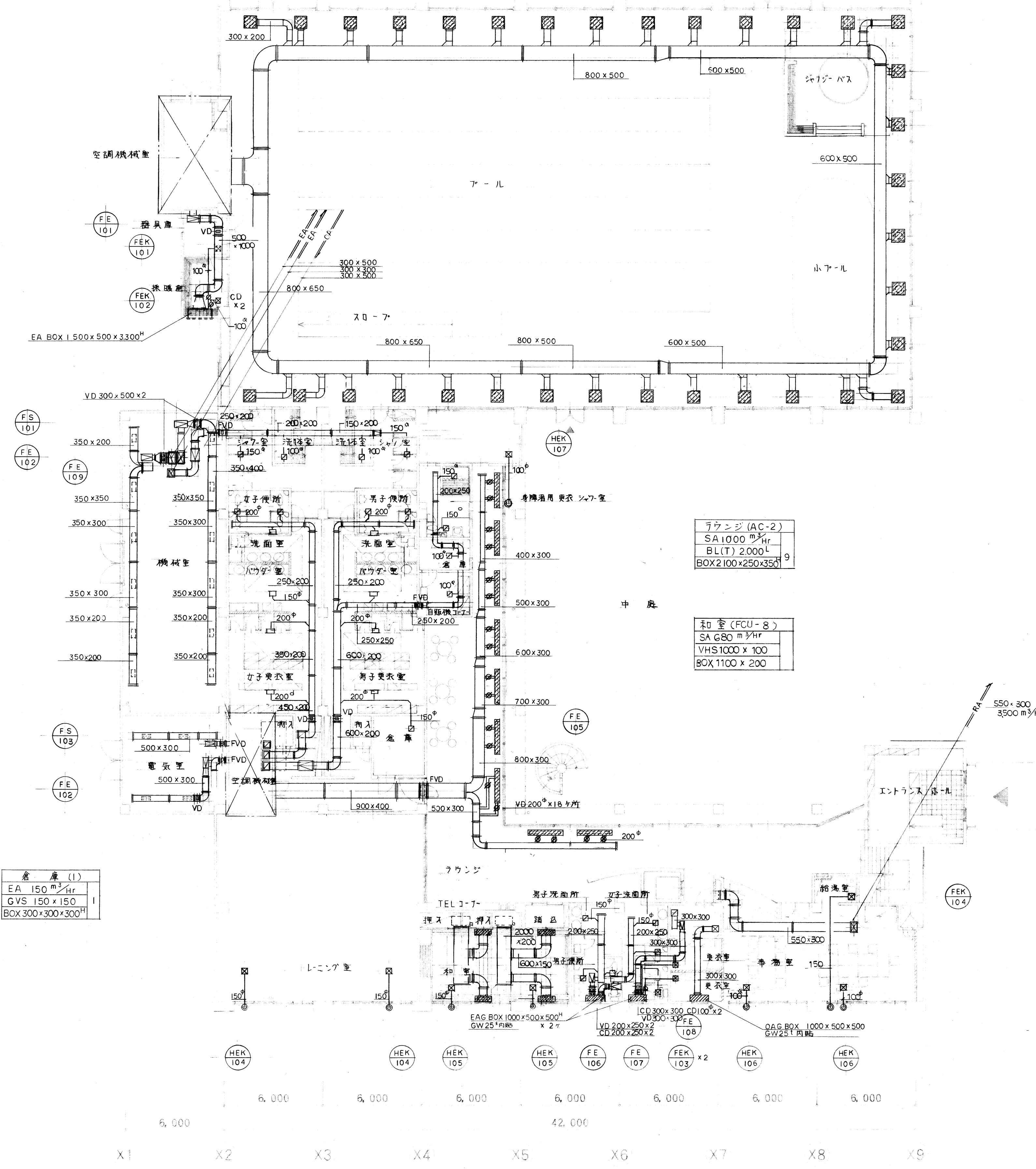
1階平面図 5=1/150
