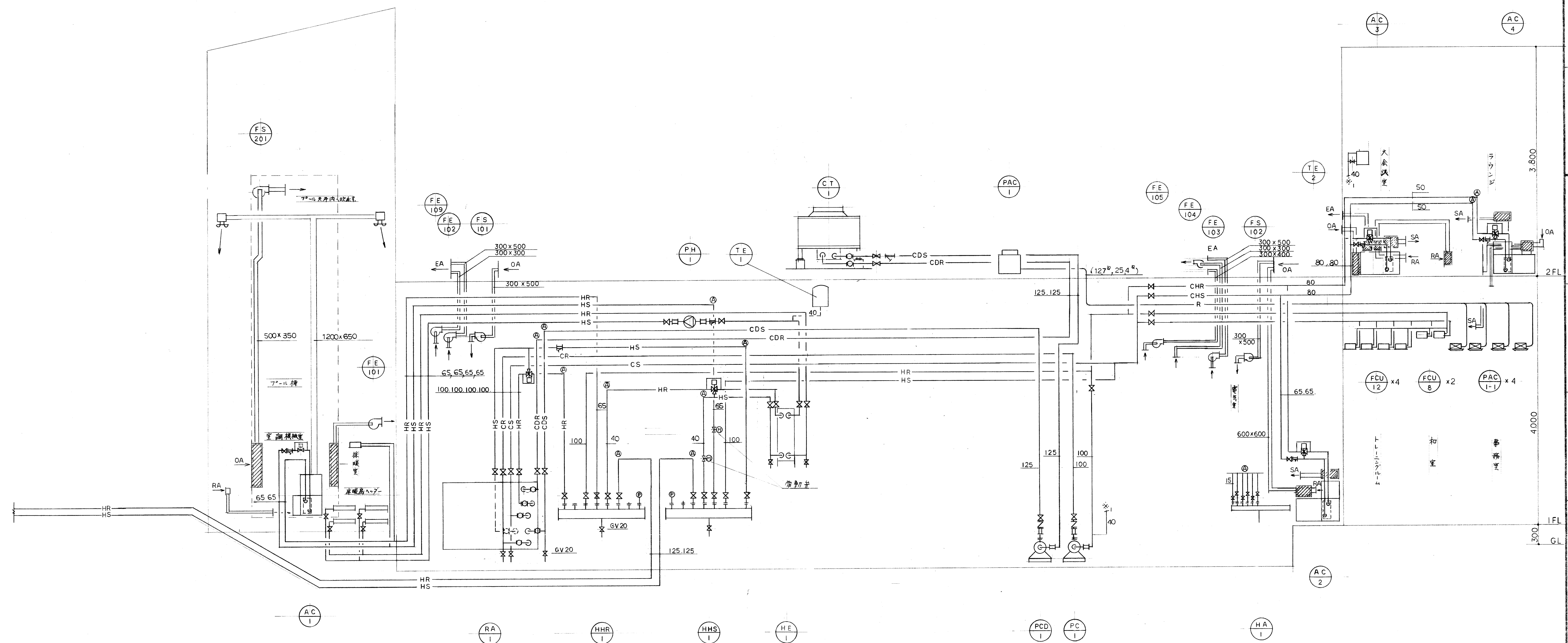
系統図(空調)
