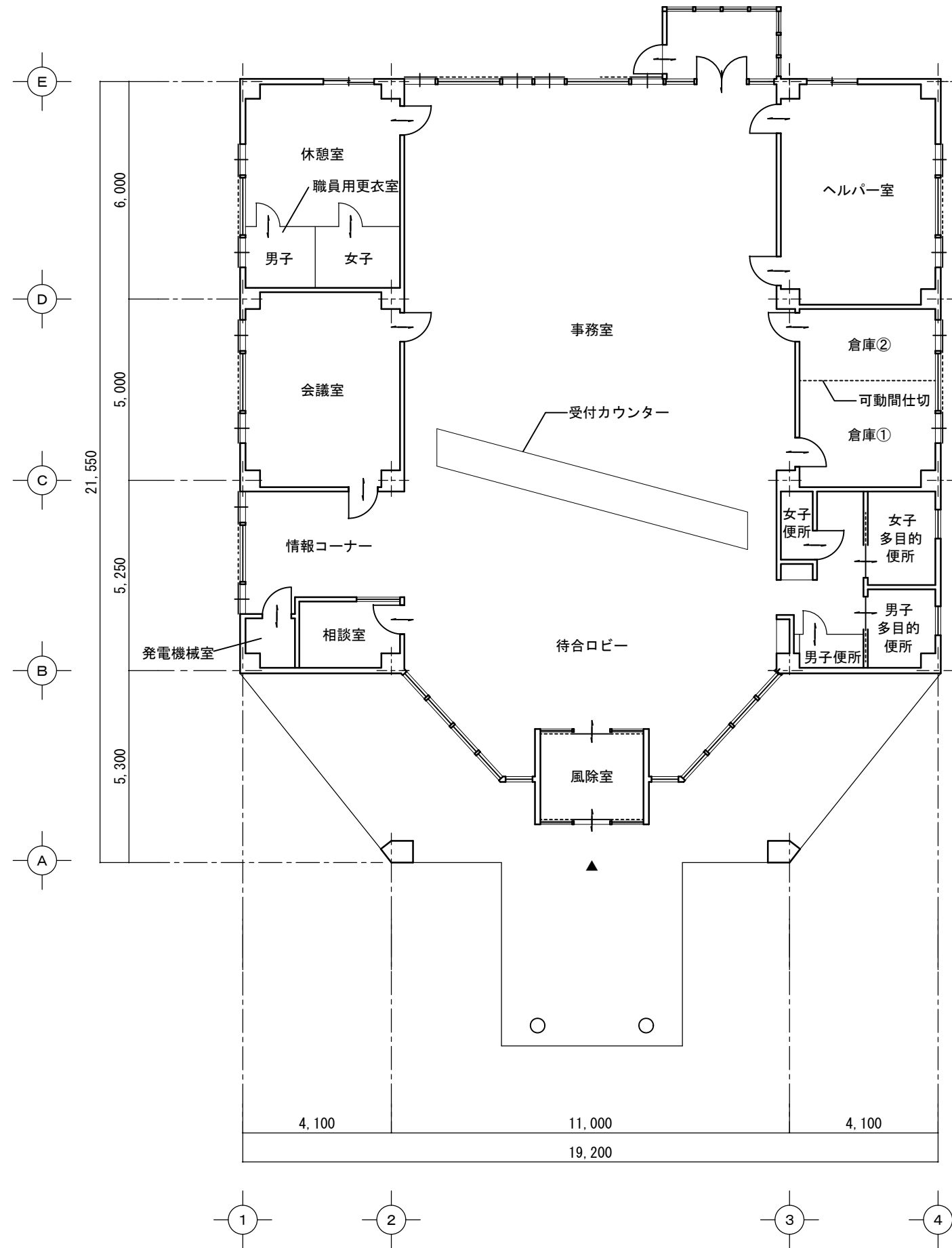
平面図 1/100
