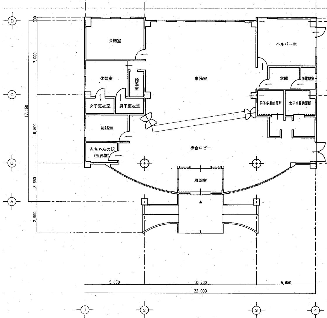
平面図 1/100
