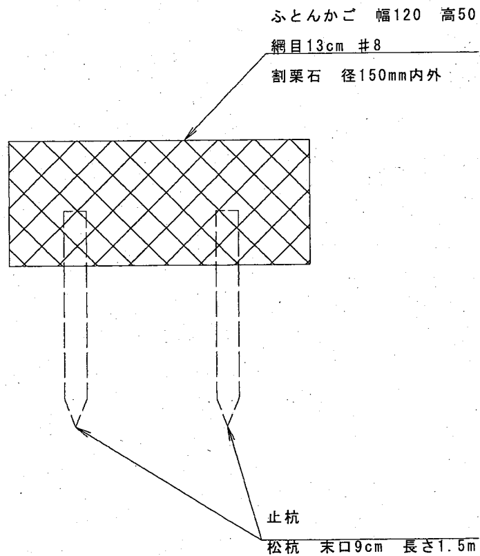
標準断面図
