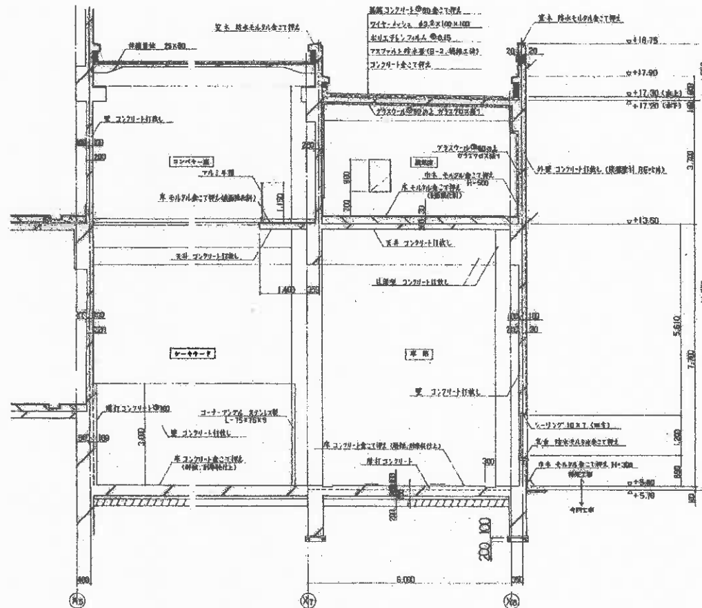
断面図 1:50
