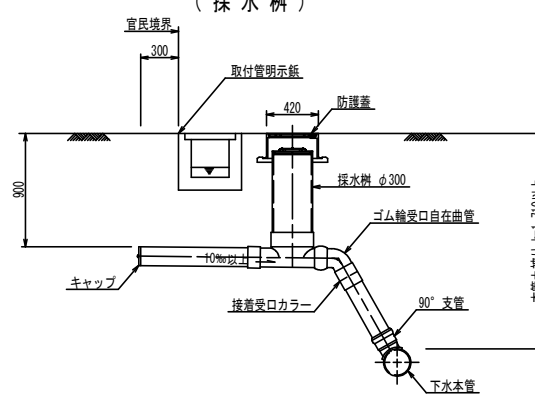
取付管掘削標準断面図 S=1:30
