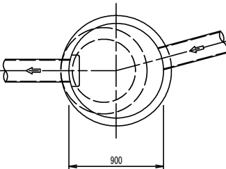
平面図 (1号)
