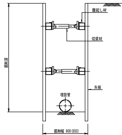
本管 矢板部 \phi 200(\phi 150)
