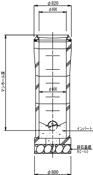
横断面図
