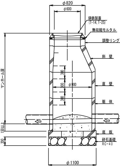
縦断面図
