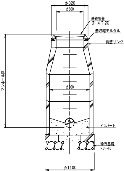
横断面図
