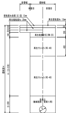
国道 (車道部 (R2000P))
