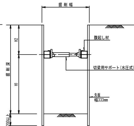
断面図②
