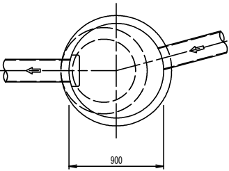
平面図 (1号)
