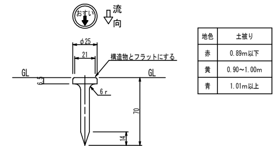
取付管位置明示板設置図 S=1:2 (その他)
