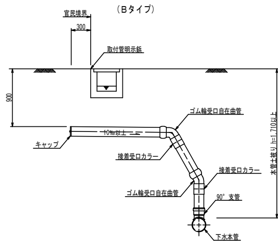
(私道部)
