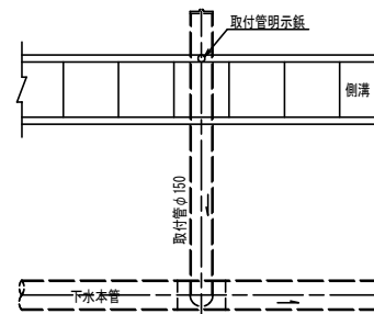
取付管位置明示鉋設置図 S=1:30 (側溝部)
