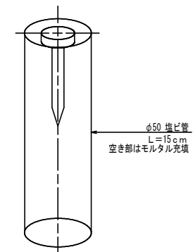
取付管位置明示板設置図 S=1:2 (その他)
