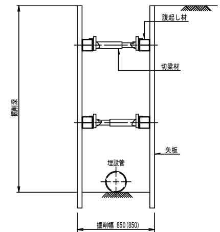
取付管 矢板部 \phi 150(\phi 100)
