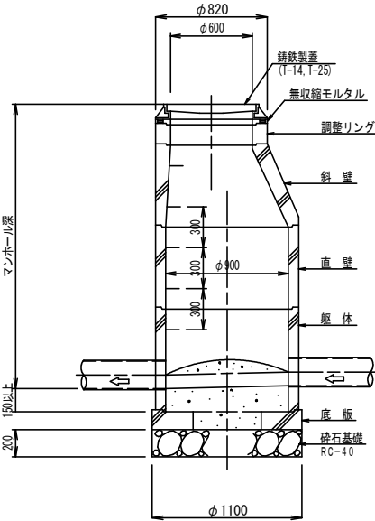
縦断面図
