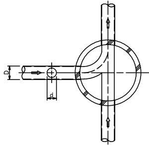
【平面図】
