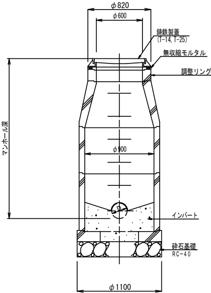
横断面図
