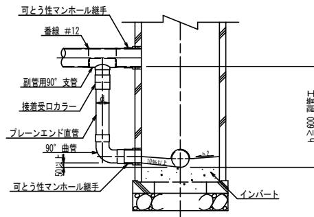
【断面図】
