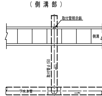
取付管位置明示板設置図 S=1:30
