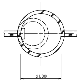
平面図 (3号)
