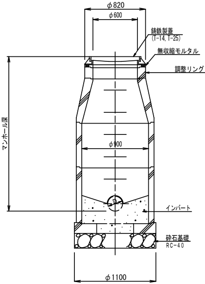
横断面図
