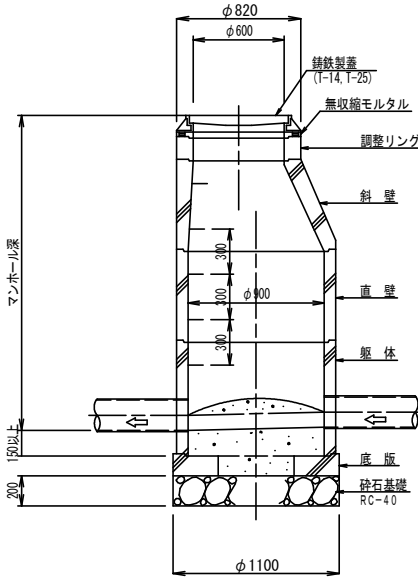
縦断面図
