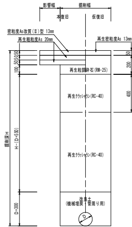
国道 (車道部 (R2000P))
