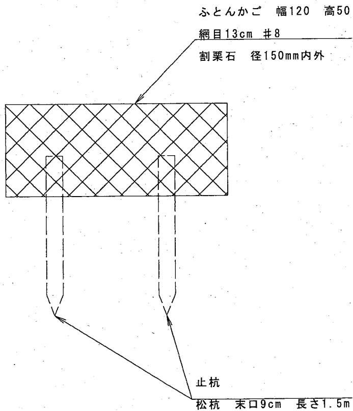
標準断面図
