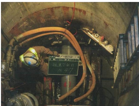
施工状況
