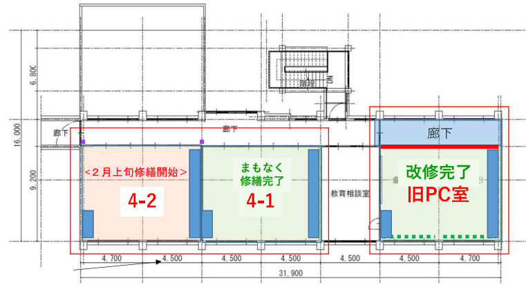
南校舎 2F 平面図
