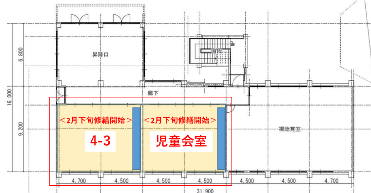
南校舎 1F 平面図
