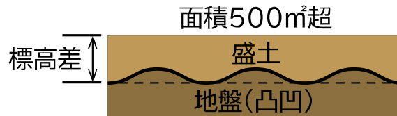
図1-10 標高差の考え方
