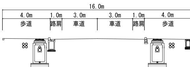
標準断面図
