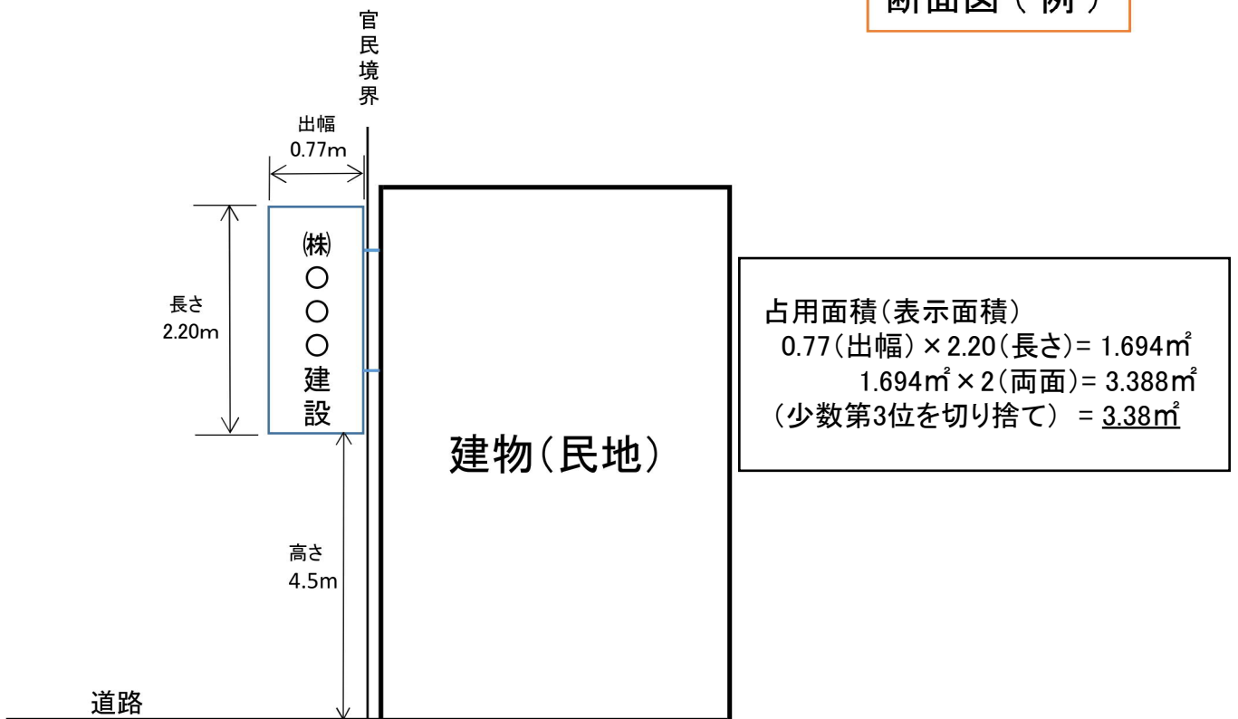
断面図(例)
