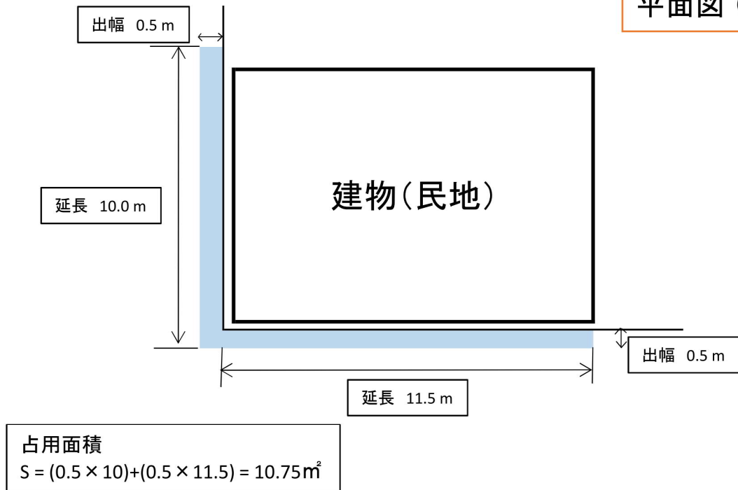
平面図(例)
