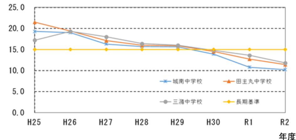
図2-1-11 PM2.5濃度経年変化
