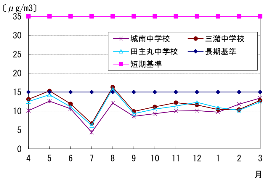
図2-1-10 令和元年度 PM2.5濃度 年間変化(月平均値)
