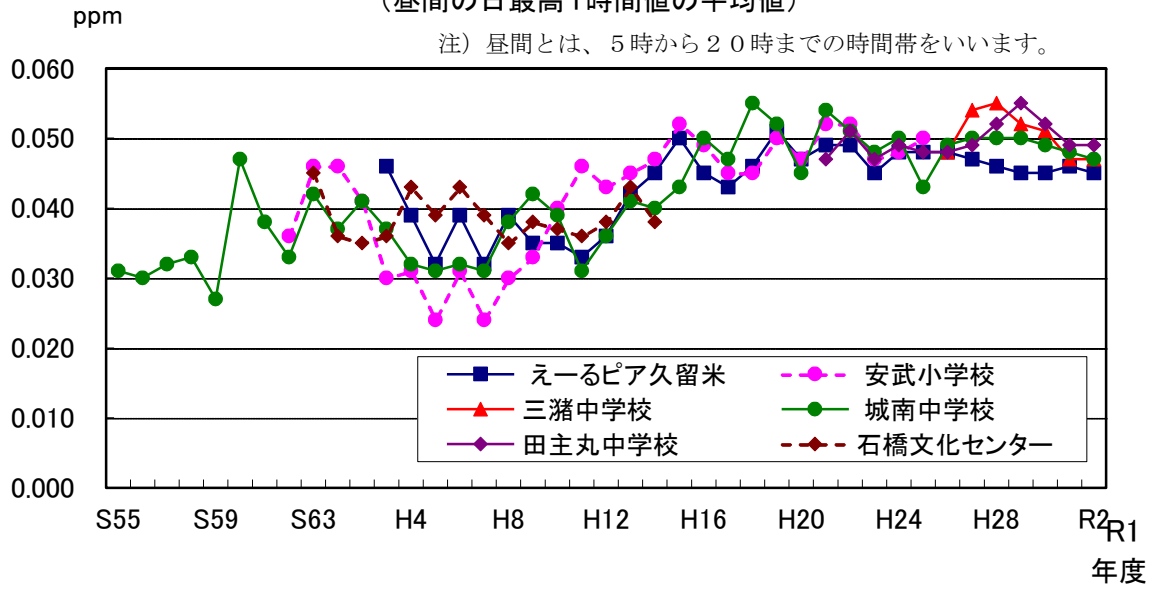
図2-1-19 光化学オキシダント 経年変化 (昼間の日最高1時間値の平均値)
