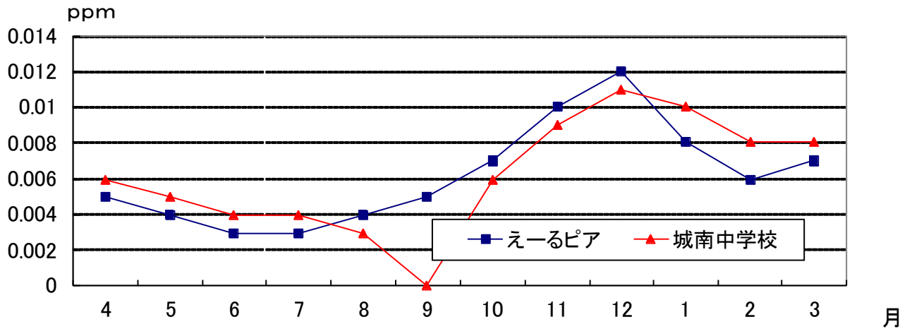
図2-1-6 令和元年度 二酸化窒素 年間変化(月平均値)
