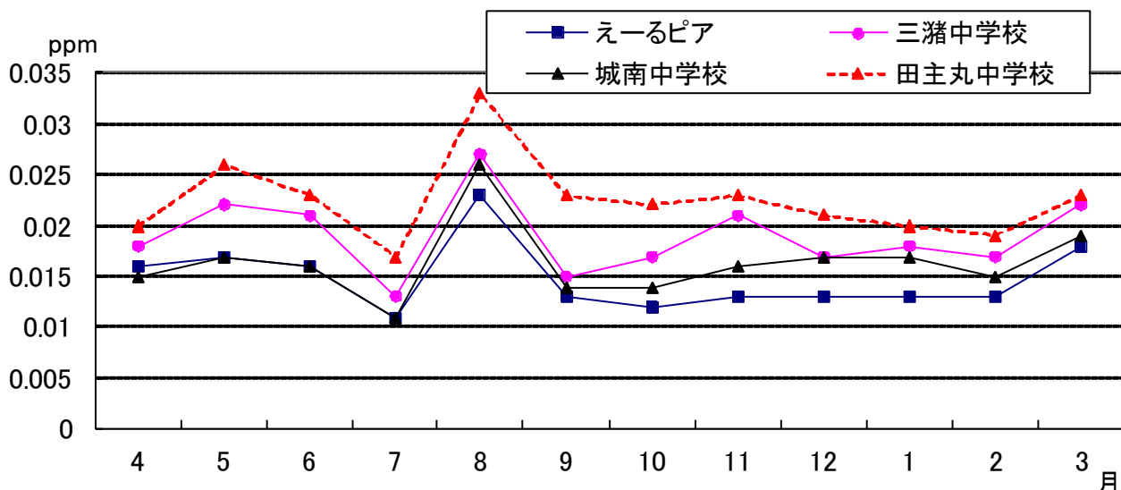
図2-1-8 令和元年度 浮遊粒子状物質 年間変化
