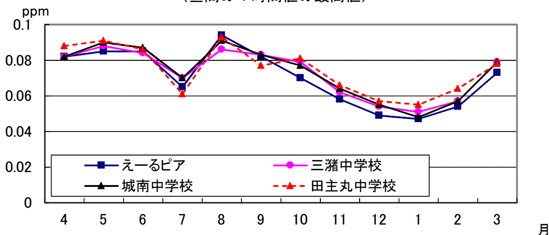
図2-1-18 令和 2 年度 光化学オキシダント年間変化 (昼間の 1 時間値の最高値)
