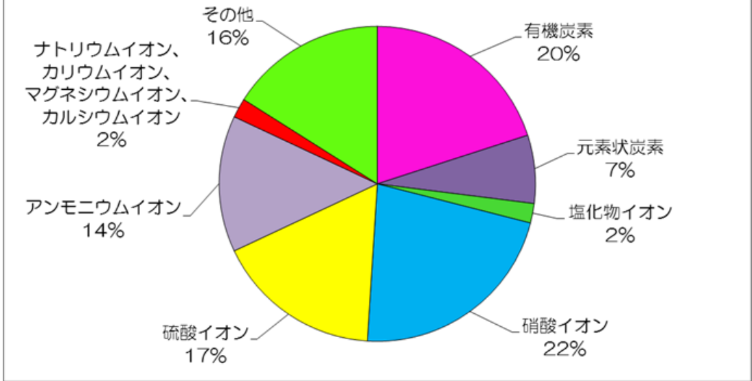
図 2-1-13 平成30年度 PM2.5 成分測定結果
