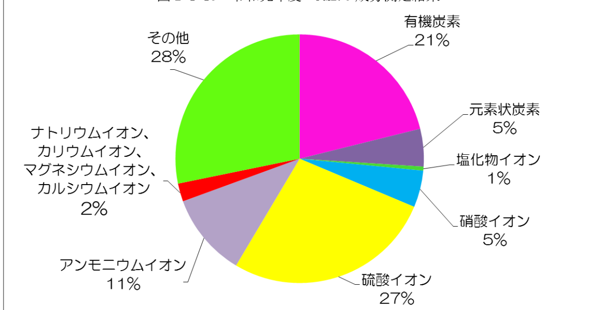
図 2-1-13 令和元年度 PM2.5 成分測定結果
