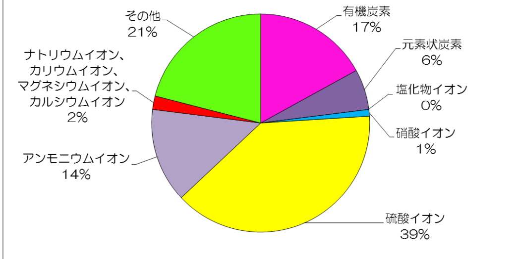
図 2-1-14 平成29年度 PM2.5 成分測定結果
