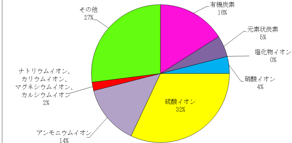
図 2-1-16 平成 27 年度 PM2.5 成分測定結果
