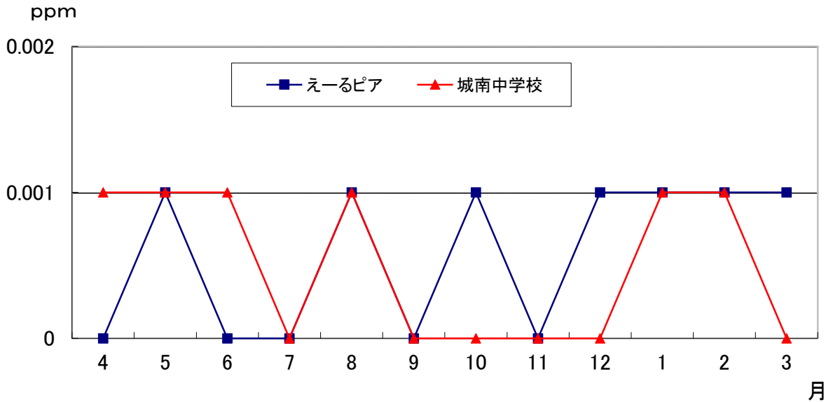
図2-1-2 令和元年度 二酸化いおう 年間変化(月平均値)
