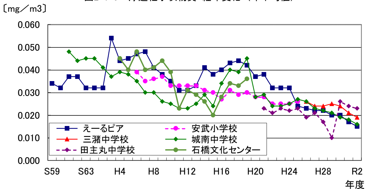
図2-1-9 浮遊粒子状物質 経年変化（年平均値）
