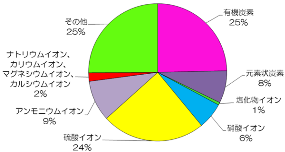
図 2-1-15 平成 28 年度 PM2.5 成分測定結果
