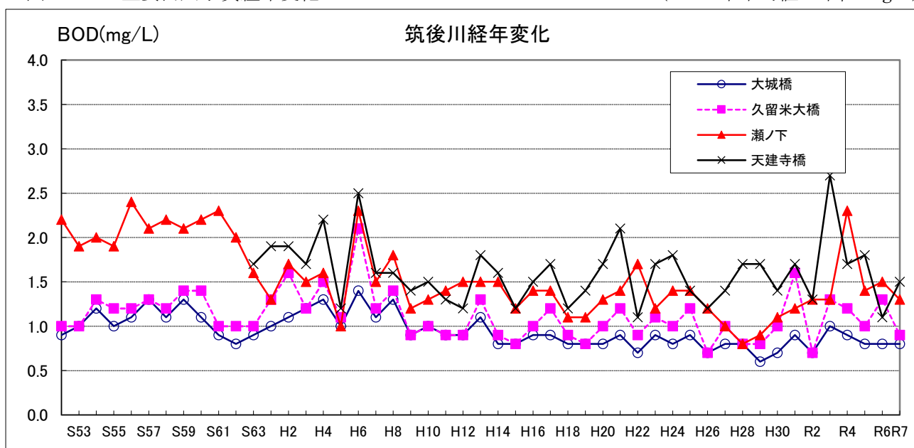
図 2-2-2 主要河川水質経年変化
