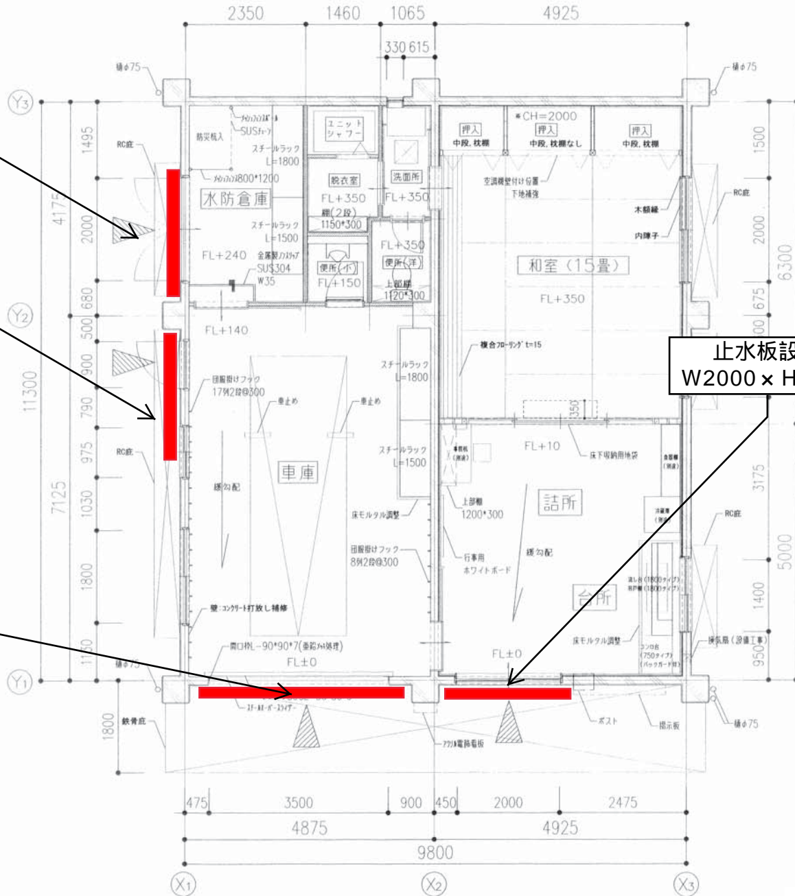
平面図 S=1:50
