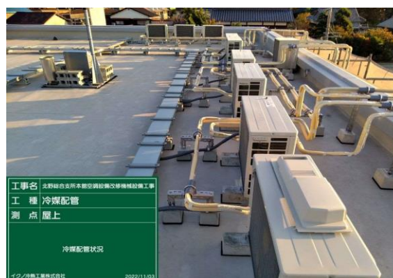
施工状況
