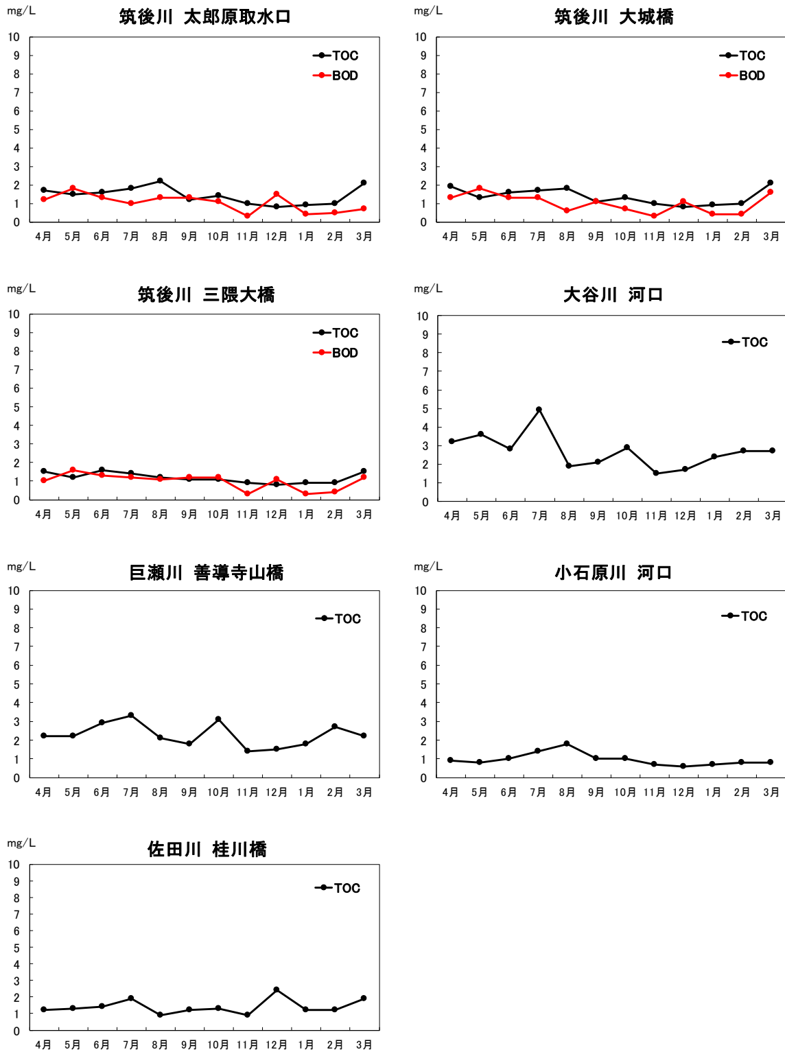
図4 生物化学的酸素要求量(BOD)、有機物質(TOC)の月変化
