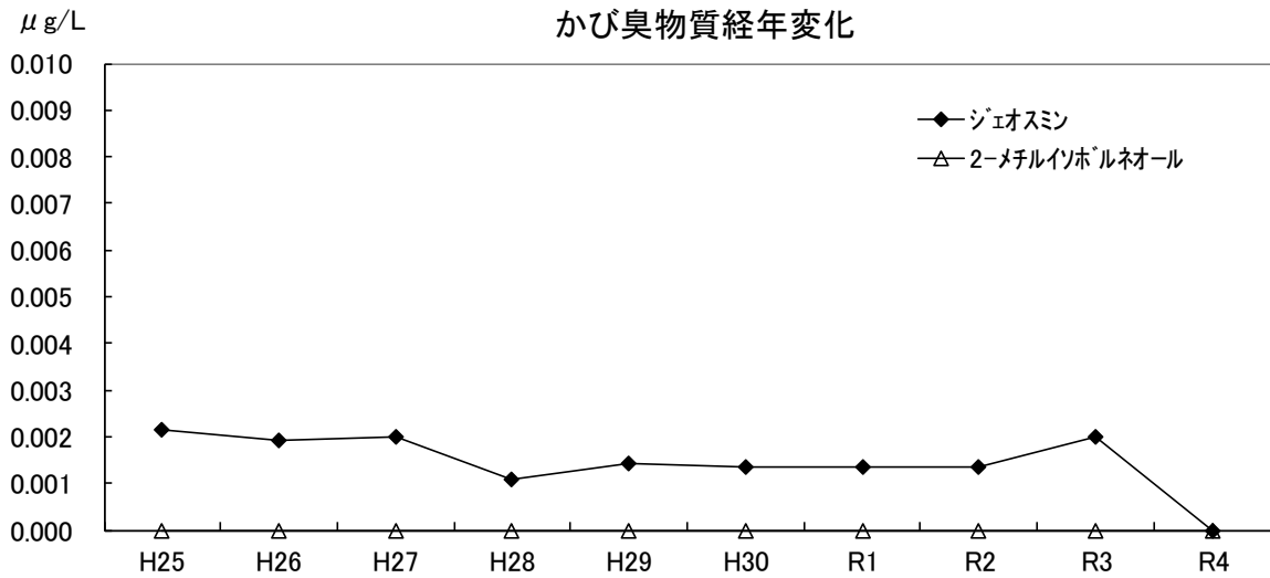
図8 筑後川太郎原取水口かび臭物質
