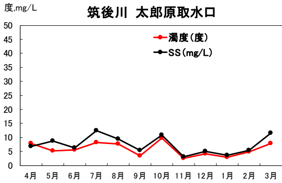
図6 濁度、SS(浮遊物質)の月変化
