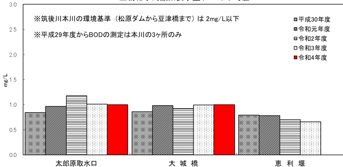
②筑後川本川水質経年変化 生物化学的酸素要求量(BOD)平均値
