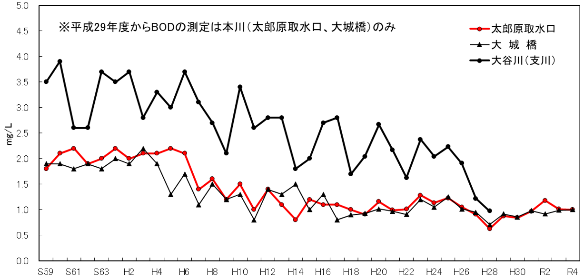
①筑後川主要地点水質経年変化 生物化学的酸素要求量(BOD)平均値
